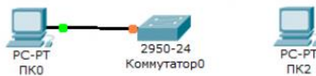
Рисунок 14- Соединение медным прямым кабелем ПК0 и коммутатор0
